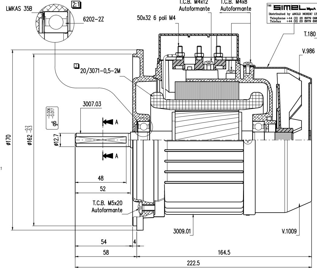
SEZ. A-A
